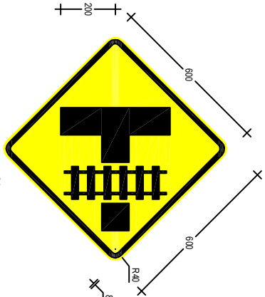
W7-12R(A) 600 x 600
